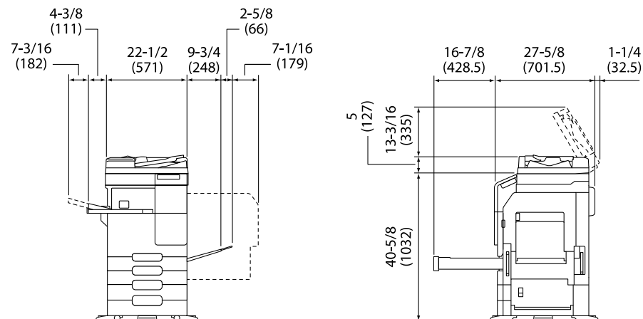
Unitatea principală + DF-633 + PC-218 + FS-533 + PK-519
